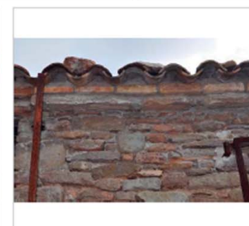
Cornisa de llosa de pedra reconstruïda. 2020 CBA
